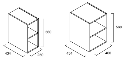
Coquetas 250 2 espacios Coquetas 400 2 espacios
