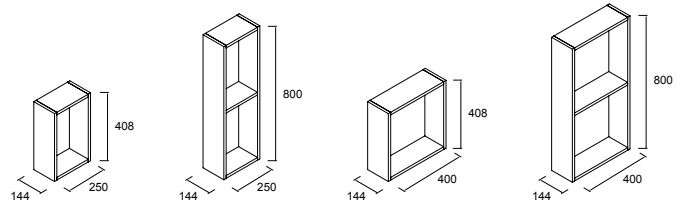
Módulo 250 1 espacio Módulo 250 2 espacios Módulo 400 1 espacio Módulo 400 2 espacios
