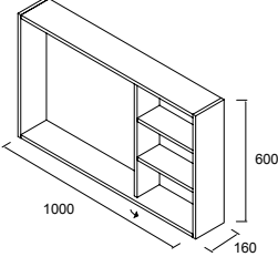
Armario PORTOBELLO 1000 1 puerta espejo con freno y luz led (4,6 W) 1000 x 600 x 160 mm
