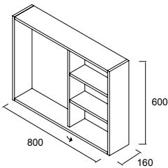
Armario PORTOBELLO 800 1 puerta espejo con freno y luz led (2,7 W) 800 x 600 x 160 mm
