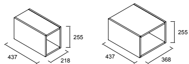
Set de 2 cubos para coqueta 250 Set de 2 cubos para coqueta 400
